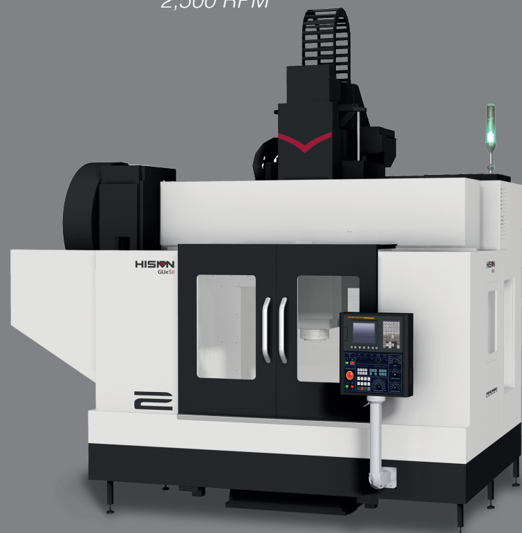
GUE5 II $3,784,924 pesos 1300mm x 700 mm x 600 mm Peso de la Máquina: 12 ton 6,000 RPM
